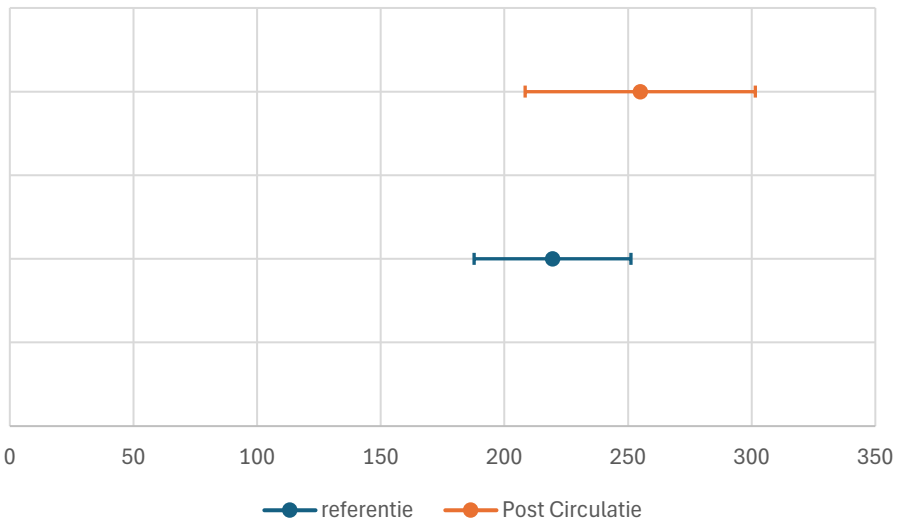
betrouwbaarheidsintervallen 2-wielers
