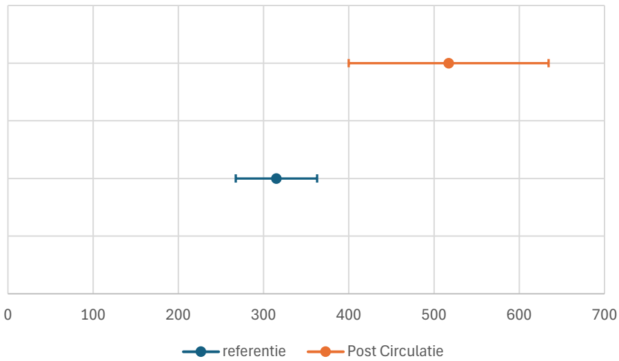
betrouwbaarheidsintervallen 2-wielers
