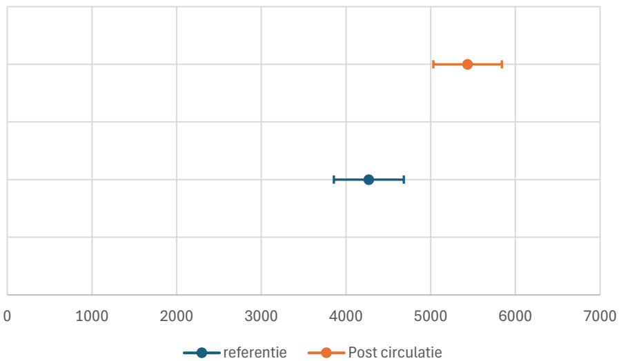
betrouwbaarheidsintervallen auto's
