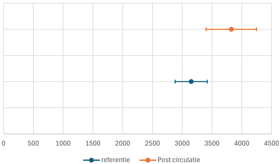
betrouwbaarheidsintervallen auto's
