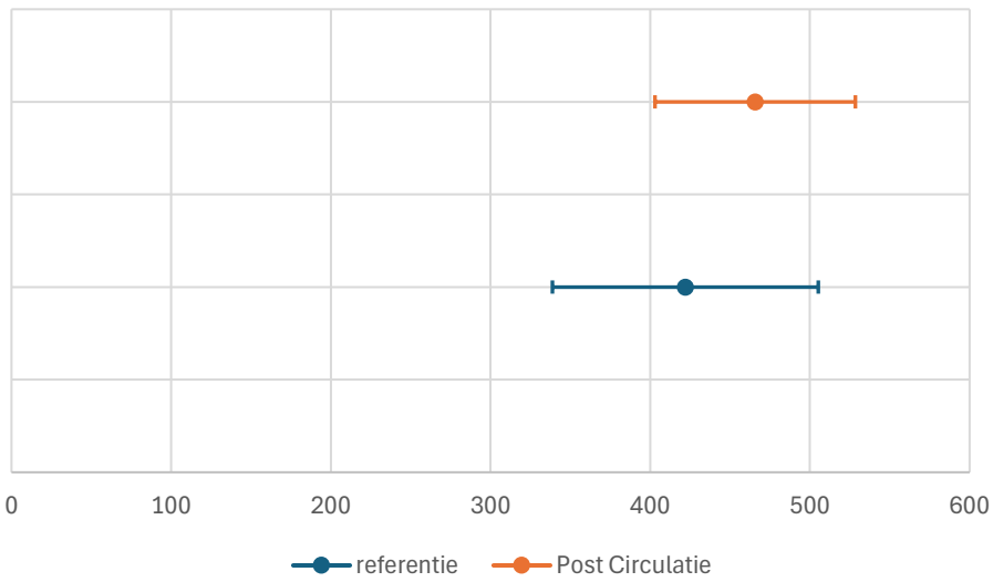
betrouwbaarheidsintervallen auto's
