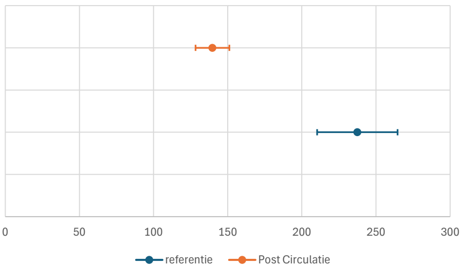
betrouwbaarheidsintervallen 2-wielers
