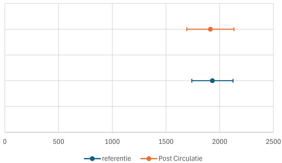
betrouwbaarheidsintervallen 2-wielers
